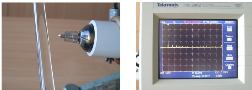
Obr. 4 Sršení náboje z nabitě skleněné tyče do hrotu sondy
