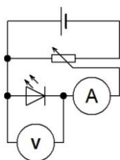
Obr. 6 Schéma obvodu
