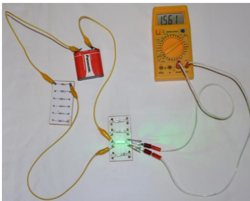
Obr. 5. Zapojený skutečný obvod
