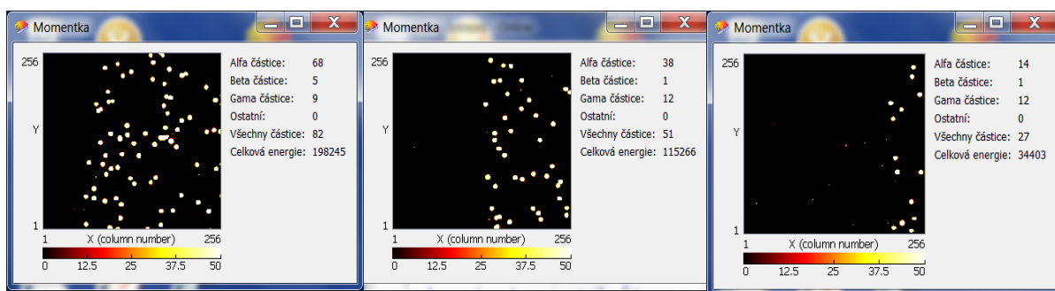
Obr. 12 - Absorpce částic alfa v kancelářském papíru.
