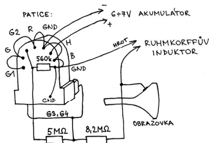
Obr. 3. Napájení obrazovky
