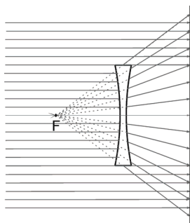
Obr. 1. Princip jednoduchého určení ohniskové vzdálenosti rozptylky
