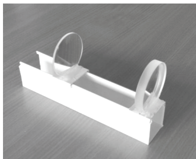
Obr. 5. Galileiho dalekohled na krátké optické lavici
