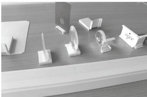
Obr. 3. Prvky jednoduché optické lavice z plastové elektroinstalační lišty
